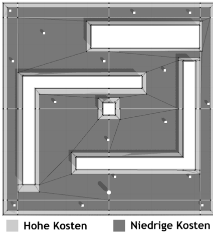
Abbildung 5: Visualisierung des gebackenen NavMeshes mit Traversierungskosten
