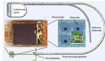
Abbildung 3: Aufbau - Subretinales Implantat [9]
