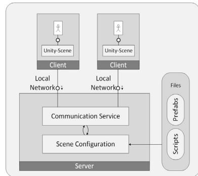
Abbildung 2: Server Client Kommunikation Block Diagramm nach FMC [3]
