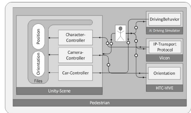
Abbildung 5: Umgesetzter Client Pedestrian
