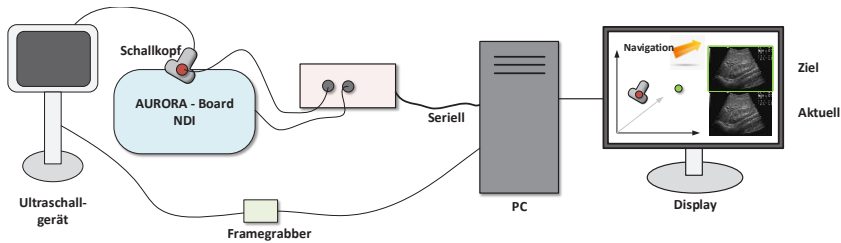
Abbildung 1 Systemaufbau mit Komponenten
