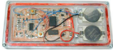
Abbildung 7: Versuchsaufbau zum Auslesen und Klonen eines 125KHz Read-Only Transponders [15]
