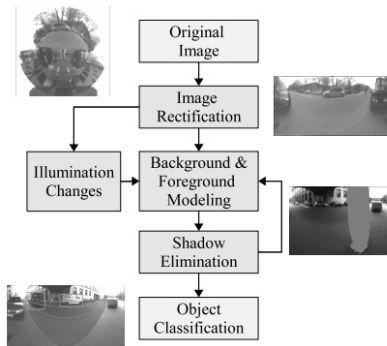
Abbildung 3: Diagramm zur Objekterkennung mit Hintergrundschätzungen, Schattenkompensation und Berücksichtigung der Beleuchtungsänderungen [14]
