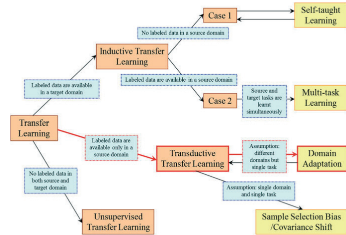
Abbildung 7: Die verschiedenen Arten des Transfer Learning [14]
