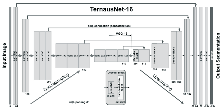
Abbildung 4: Architektur des TerausNet-16 [12]
