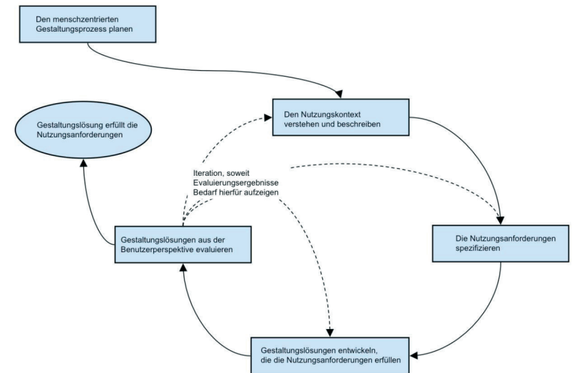
Abbildung 3: Schematische Darstellung des menschenzentrierten Designprozesses nach ISO 9241-210 [17]
