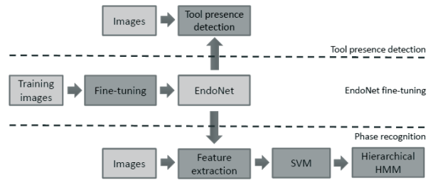
Abbildung 6: Gesamtarchitektur des Ansatzes von [5]
