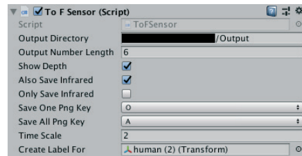
Abbildung 4: Das ToF Sensor Script und dessen Parameter
