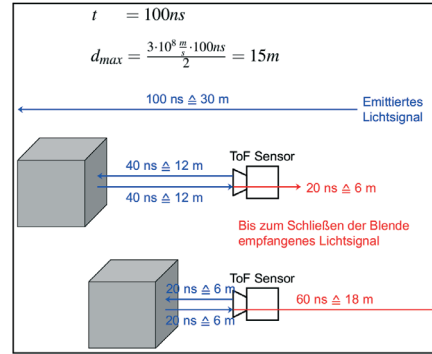
Abbildung 1: Vereinfachte Darstellung der Funktionsweise eines ToF Sensors mit Pulse Modulation
