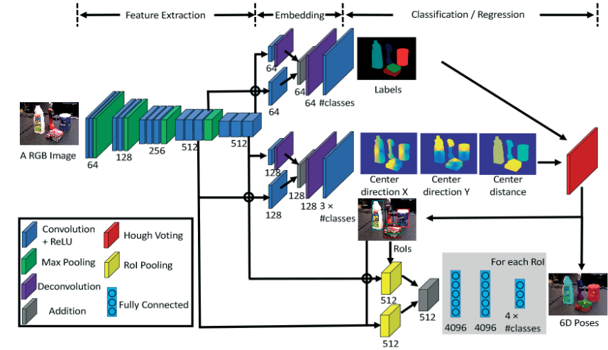
Abbildung 3: Architektur von PoseCNN für die 6D-Object Pose Estimation. [14]
