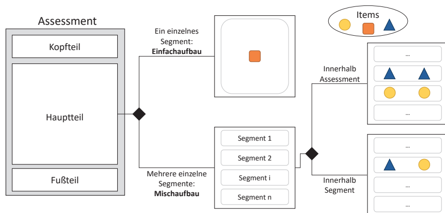
Abbildung 3: Schematischer Aufbau eines Assessments
