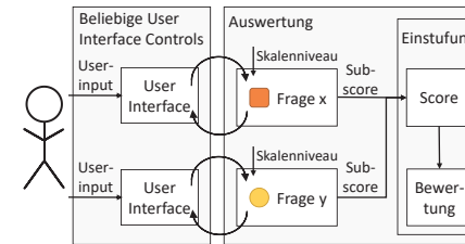
Abbildung 9: Softwaremodellierung bei Auswertearithmetik „gewichteter Score“
