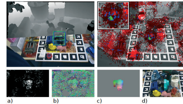
Abbildung 2: Die Methode von Brachmann et al. [10] ist in der Lage, die richtige Pose zu finden, in der eine Template-basierte Methode versagt. Das Testbild (a) zeigt eine Situation mit starker Okklusion. Die Pose Estimation (Posenschätzung) von diesem Ansatz ist blau dargestellt. Die Pose, die durch die Neuimplementierung der Methode von Hinterstoisser et al. aus [26] dargestellt wird, ist rot. (b) Die Koordinatenvorhersagen für (a) aus einem Baum, der dem RGB-Würfel zugeordnet und mit p_c, i multipliziert wurde. (c) Ground Truth Objektkoordinaten für eine Abbildung auf den RGB-Würfel. (d) Testbild mit extremen Lichtverhältnissen, die sich vom Trainingsset unterscheiden. Geschätzte Posen werden wie in (a) angezeigt. [10]
