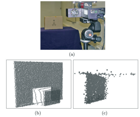
Abbildung 3: Flying Pixels Effekt [5]
