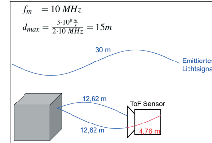
Abbildung 2: Vereinfachte Darstellung der Funktionsweise eines ToF Sensors mit CWIM
